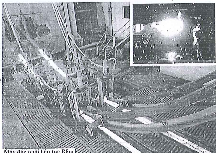
Máy đúc phôi liên tục R8m
